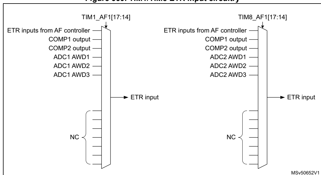
Figure 339. TIM1/TIM8 ETR input circuitry
