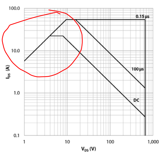
GS66506T I_{DS} - V_{DS} SOA
